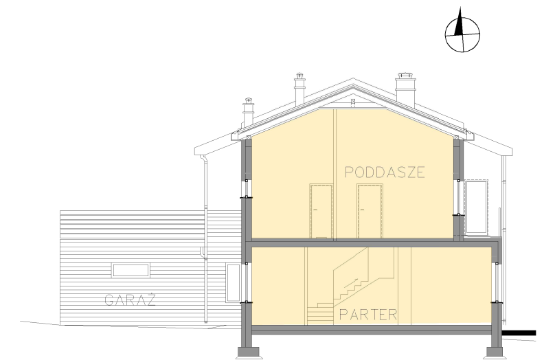
PRZEKRÓJ A'-A'
